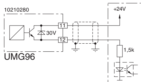
Abb. Verwendung als Impulsausgang auf Optokoppler
