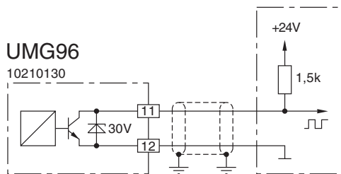
Abb. Verwendung als Impulsausgang
