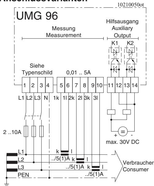
Abb.: Anschlussbeispiel 1 Vierleitermessung mit drei Stromwandlern.
