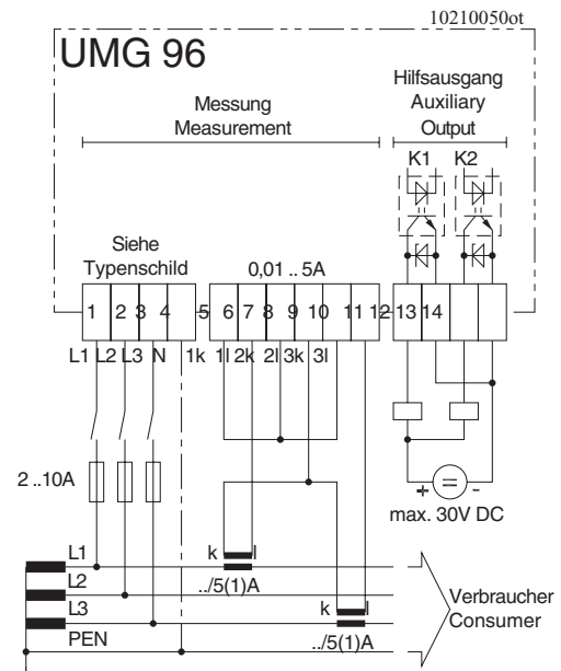
Abb.: Anschlussbeispiel 2 Vierleitermessung mit zwei Stromwandlern.
