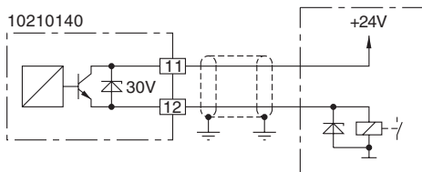
Abb. Schaltausgang mit externem Relais im Minus.
