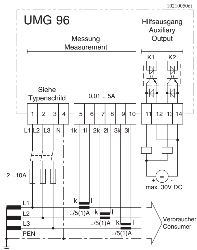
Abb.: Anschlussbeispiel, Vierleitermessung mit drei Stromwandlern
