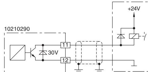
Abb. Schaltausgang mit externem Relais im Plus.
