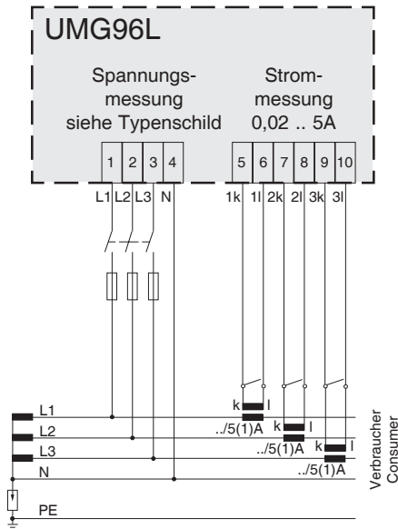
Abb.: Anschlussbeispiel 7 Messung im IT-Netz über drei Stromwandler.
