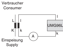
Abb. Anschlussbeispiel: UMG96L mit Ampere-meter in Reihe.
