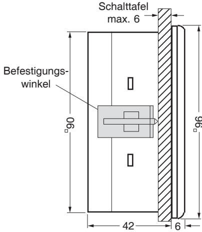
Abb. Seitenansicht
