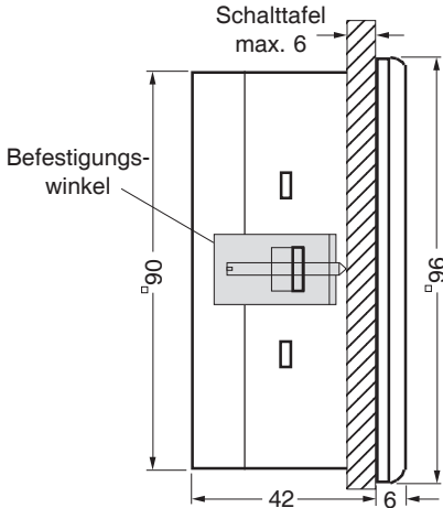
Abb. Seitenansicht
