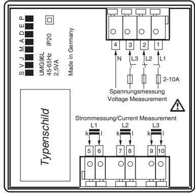
Abb. Rückseite
