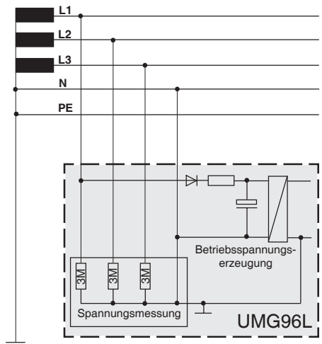
Abb. Betriebsspannungsgewinnung aus der Messspannung.
