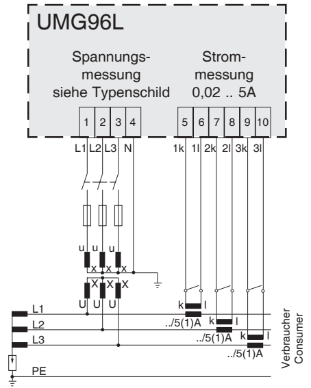
Abb.: Anschlussbeispiel 8 Messung im IT-Netz mit drei Spannungswandlern und drei Stromwandlern.
