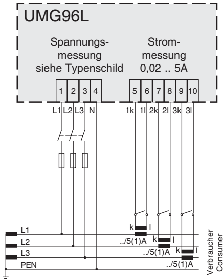
Abb.: Anschlußbeispiel 1 Vierleitermessung mit drei Stromwandlern.
