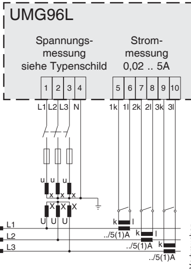
Abb.: Anschlussbeispiel 5 Mittelspannungsseitige Messung mit drei Spannungswandlern und drei Stromwandlern.
