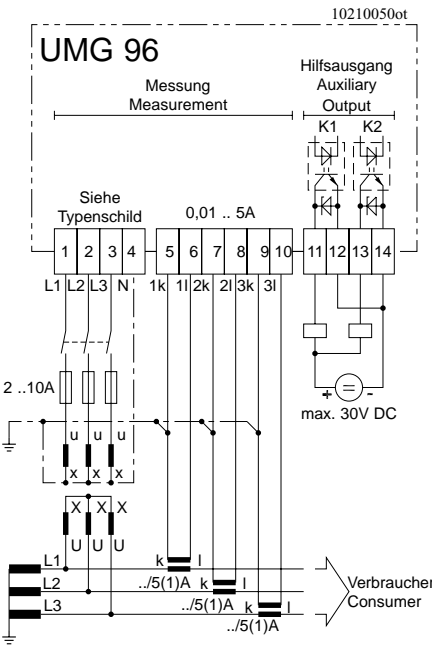
Abb.: Anschlussbeispiel 3 Dreileitermessung mit Spannungswandlern und drei Stromwandlern.
