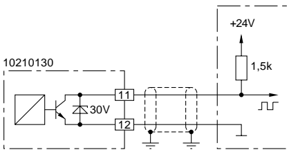
Abb. Verwendung als Impulsausgang
