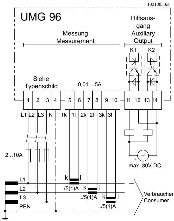
Abb.: Anschlussbeispiel, Vierleitermessung mit drei Stromwandlern
