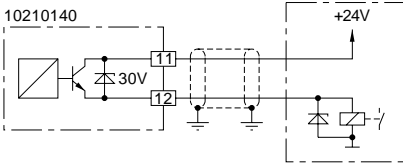
Abb. Schaltausgang mit externem Relais im Minus.
