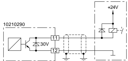
Abb. Schaltausgang mit externem Relais im Plus.
